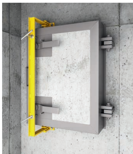
SRT Schwenkbügel für Notausstieg
